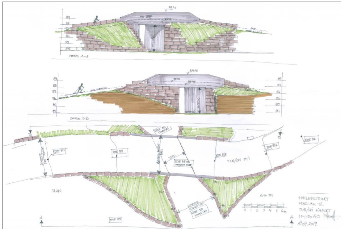
Ill 28: Tidligere planlagt viadukt/kulvert utgår av planforslaget og skiløype (o_BST) blir liggende i terrenget gjennom hele planområdet.
