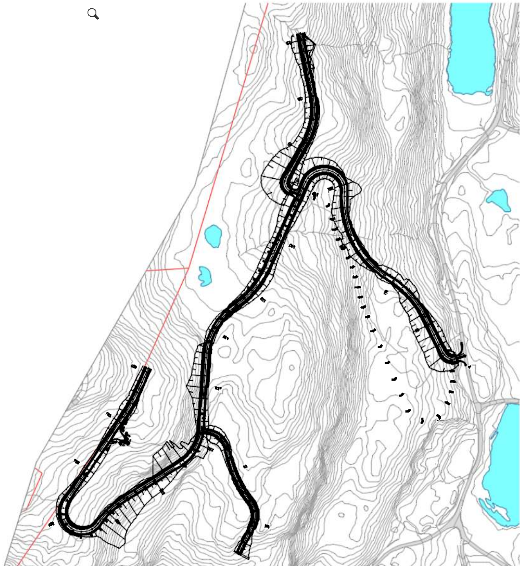
Figur 3-6 Vegprofil for vei 8, 10 og 11 innefor felt D.
